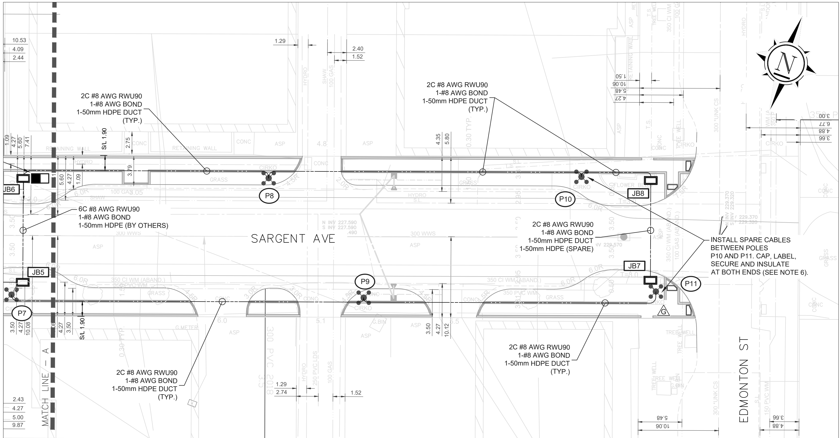
PLAN 1:250
